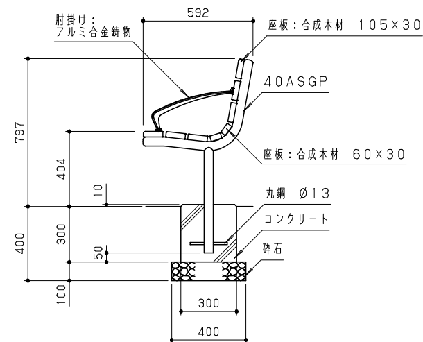
側面図 S = 1 / 20
