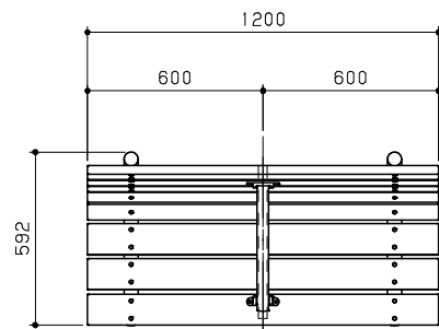
平面図 S = 1 / 20
