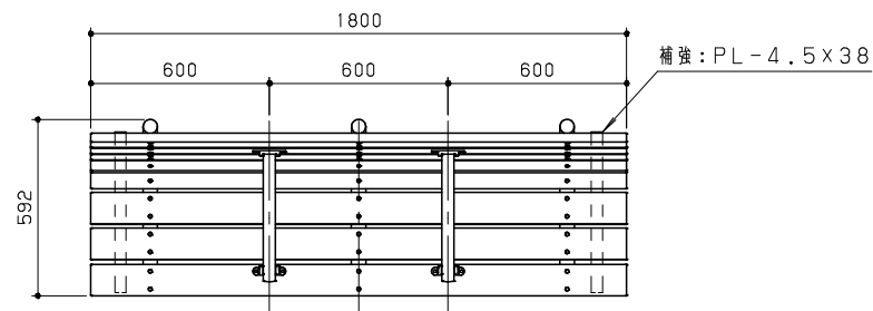
平面図 S = 1 / 20
