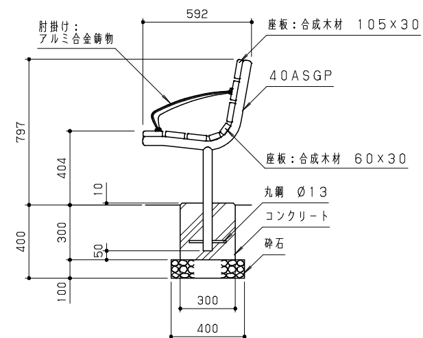
側面図 S = 1 / 20
