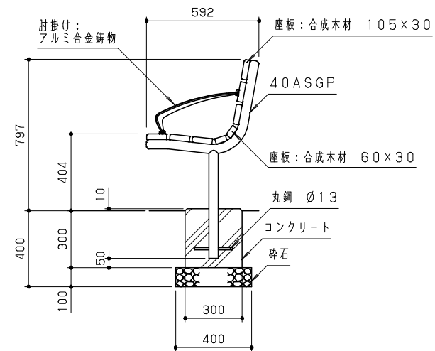
側面図 S = 1 / 20
