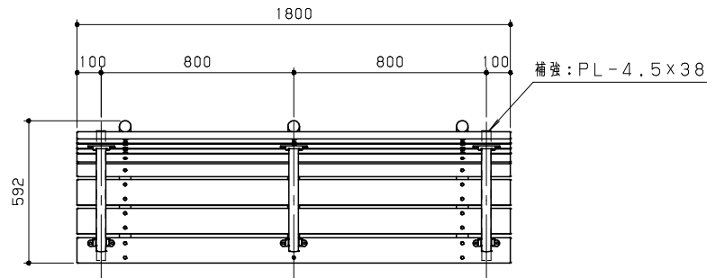
平面図 S = 1 / 20
