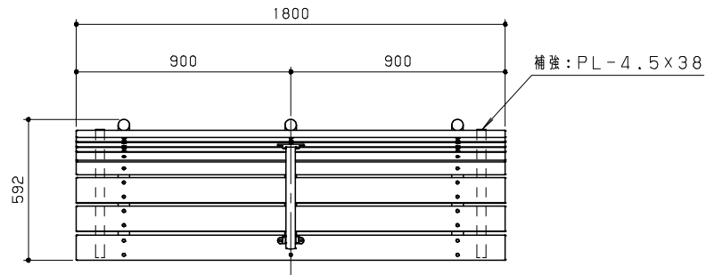
平面図 S = 1/20
