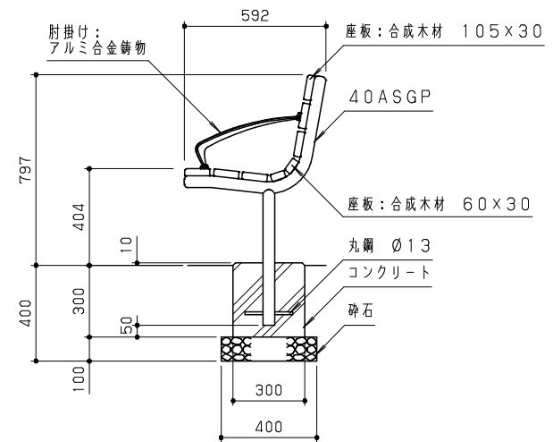
側面図 S = 1/20
