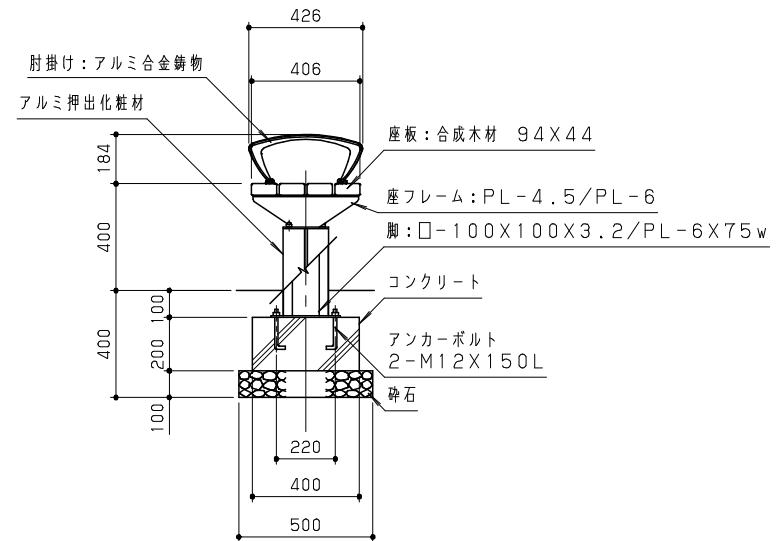
側面図 S = 1 / 20
