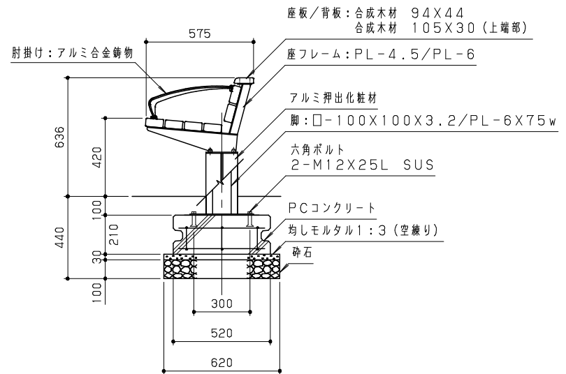
側面図 S = 1 / 20
