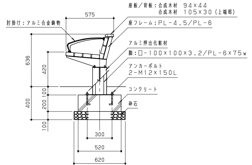
側面図 S = 1 / 20
