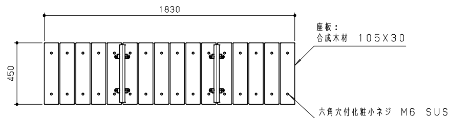
平面図 S = 1 / 20
