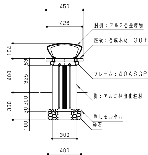
断面図 S = 1 / 20
