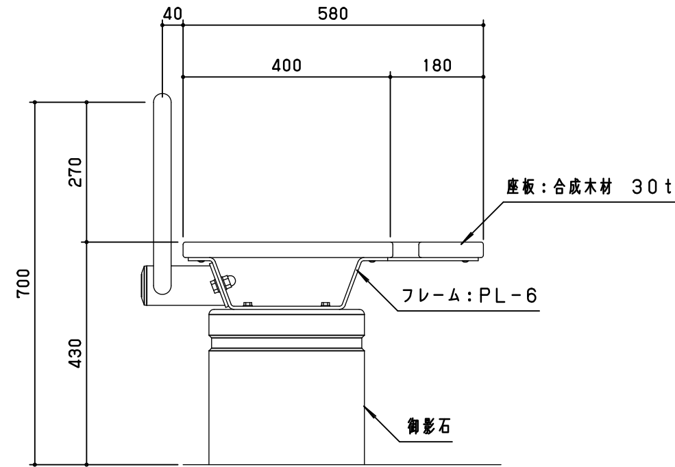
正面図 S = 1 / 10
