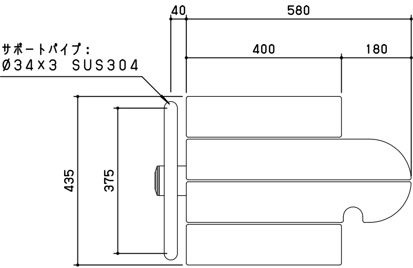
平面図 S = 1 / 10
