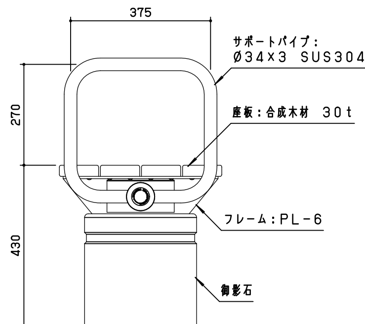
左側面図 S=1/10
