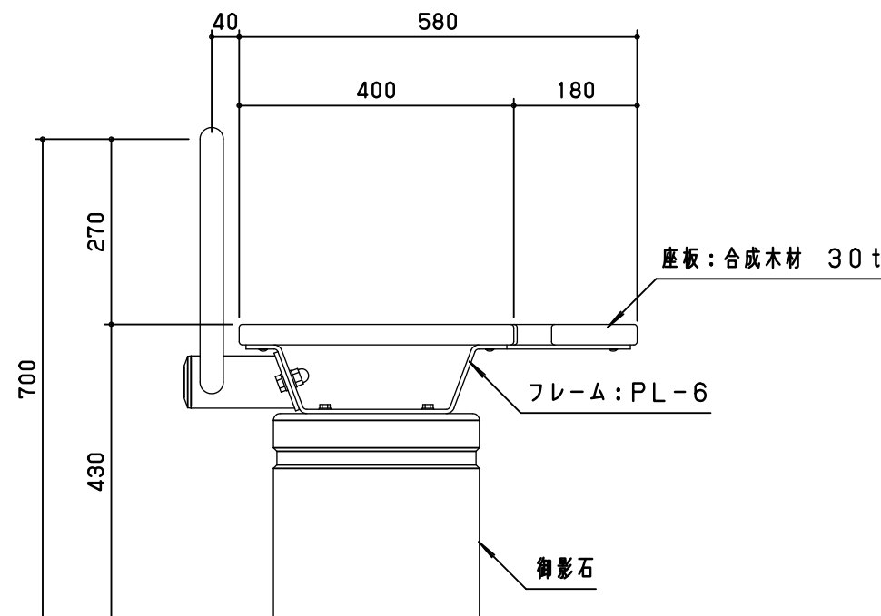
正面図 S=1/10
