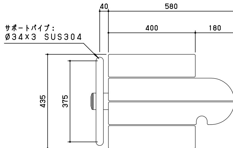
平面図 S=1/10
