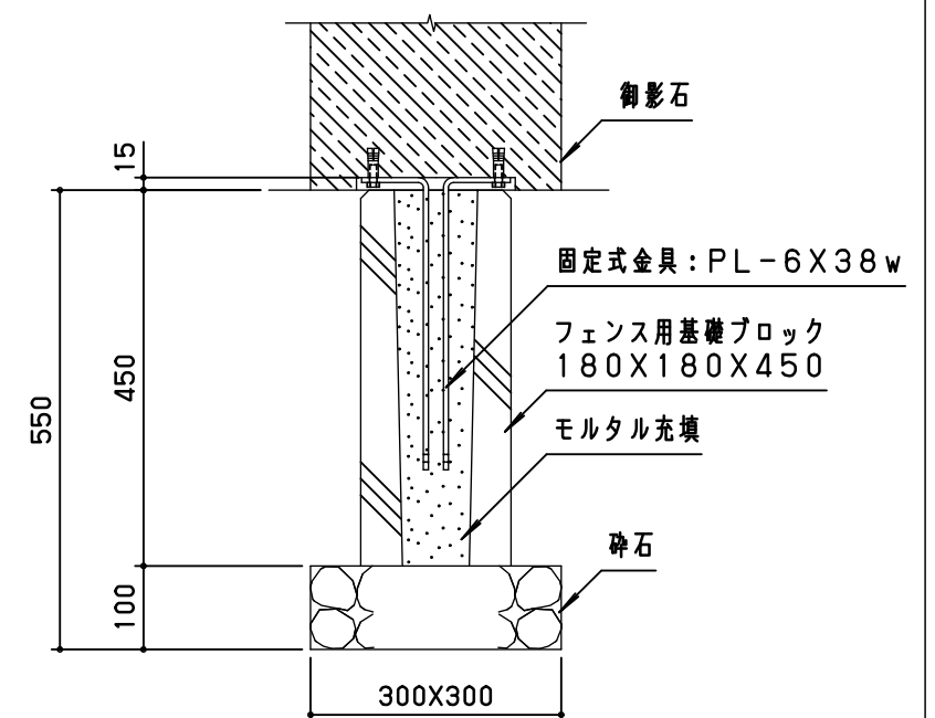
基礎詳細図 S=1/10
