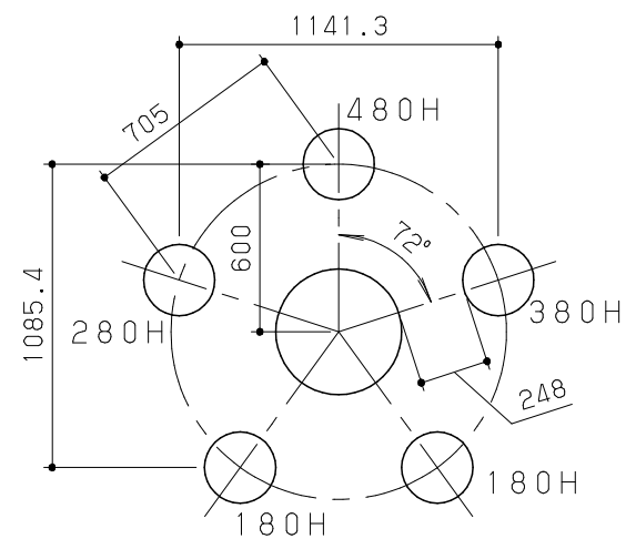
平面図 S = 1 / 30
