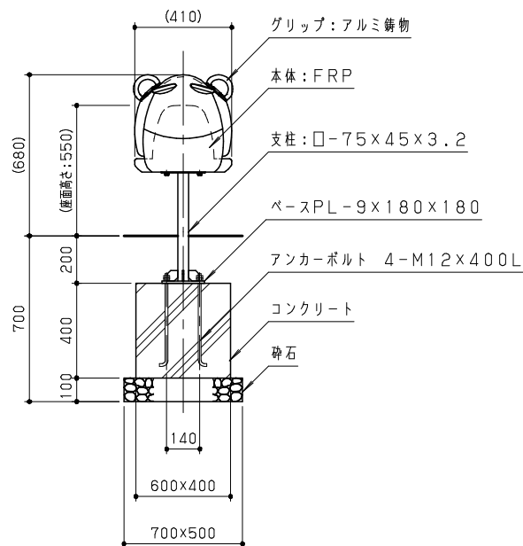
側面図 S=1/20
