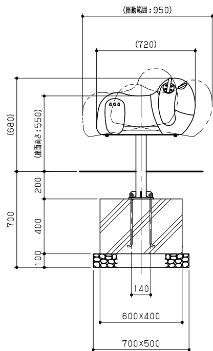
立面図 S=1/20
