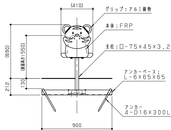
側面図 S=1/20
