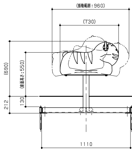
立面図 S=1/20
