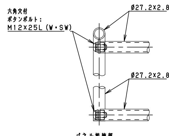
パネル接続部 詳細図 S = 1 / 5
