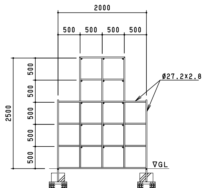
立面図 S = 1 / 50
