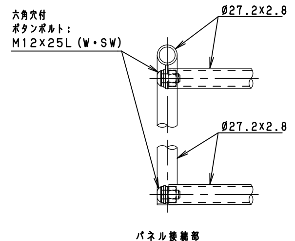
パネル接合部 詳細図 S=1/5
