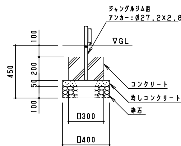
基礎断面詳細図 S=1/20
