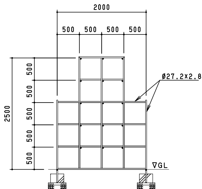
立面図 S=1/50
