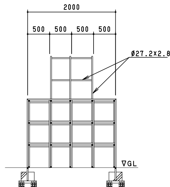
側面図 S=1/50
