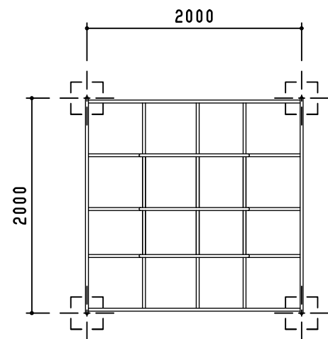
平面図 S=1/50
