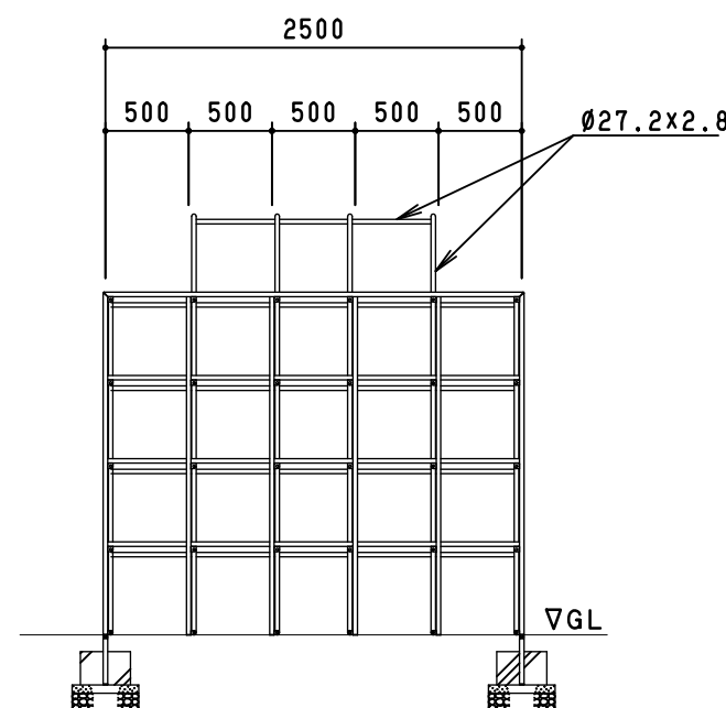
側面図 S = 1 / 50
