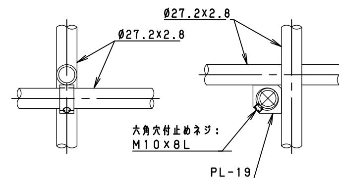
止めネジジョイント部
