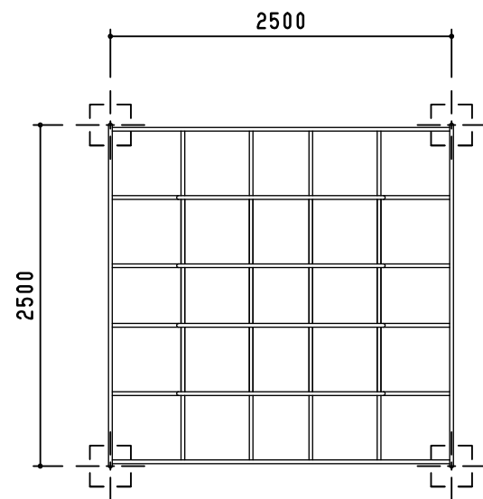
平面図 S = 1 / 50
