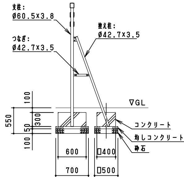
側面図 S=1/50
