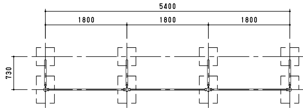
平面図 S=1/50
