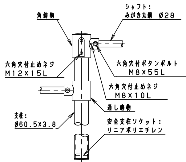
鋳物部/柱脚部詳細図 S=1/10
