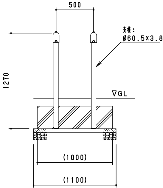
側面図 S = 1 / 30
