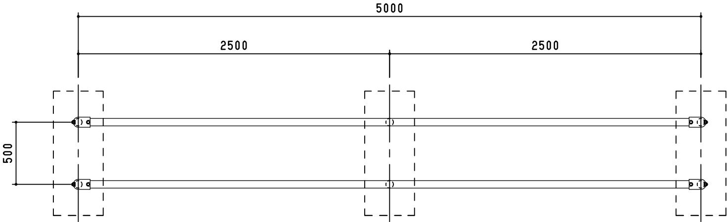
立面図 S = 1 / 30
