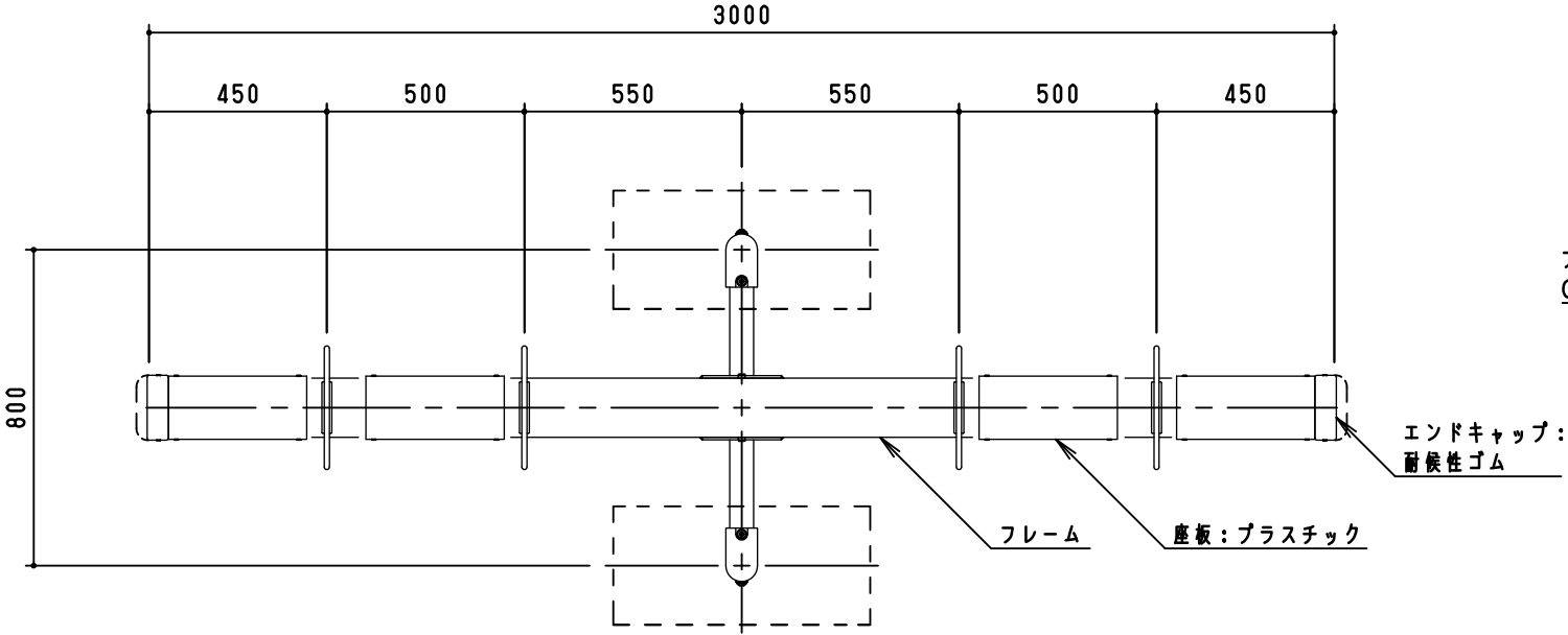
平面図 S = 1 / 20
