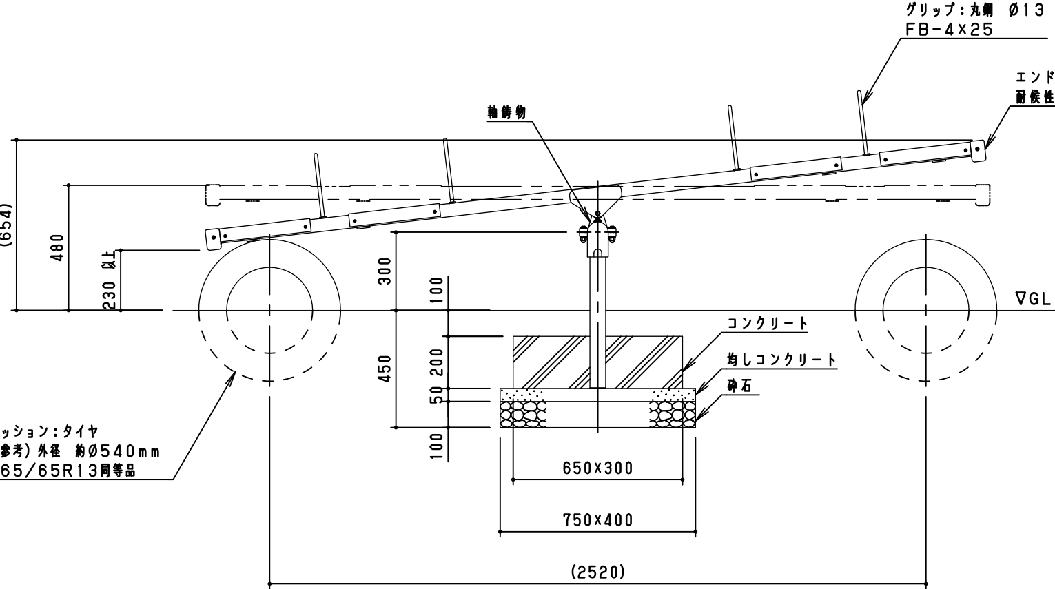
立面図 S = 1 / 20
