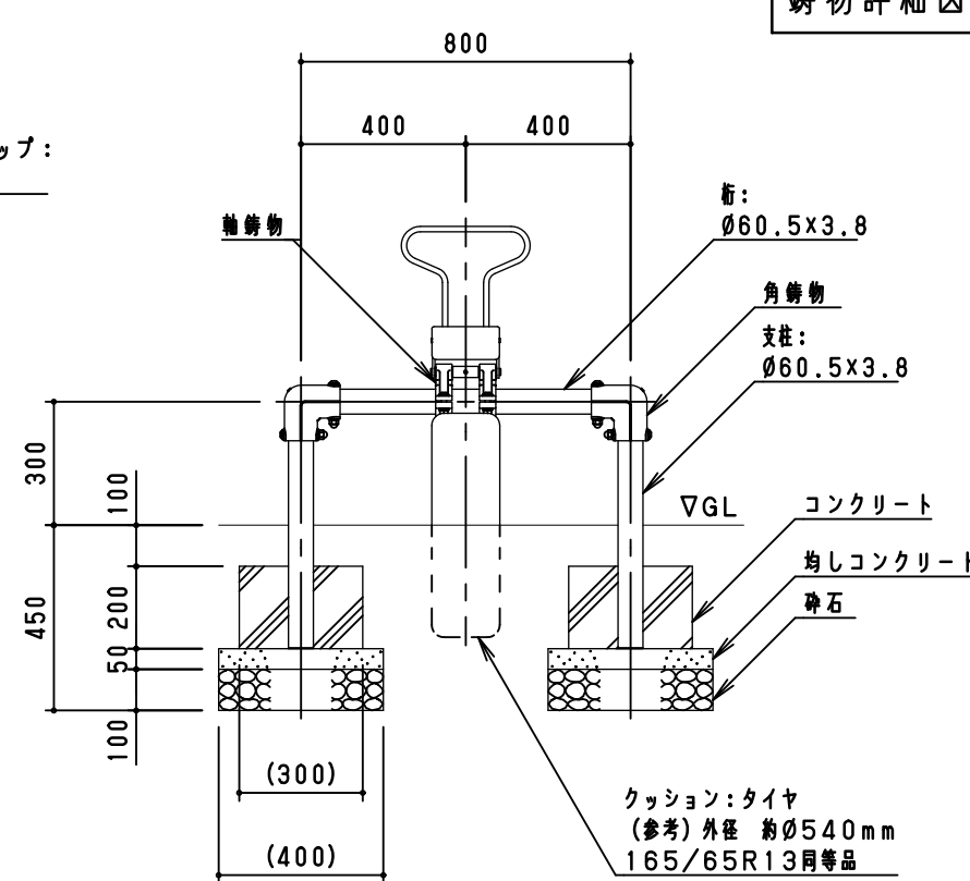
側面図 S = 1 / 20
