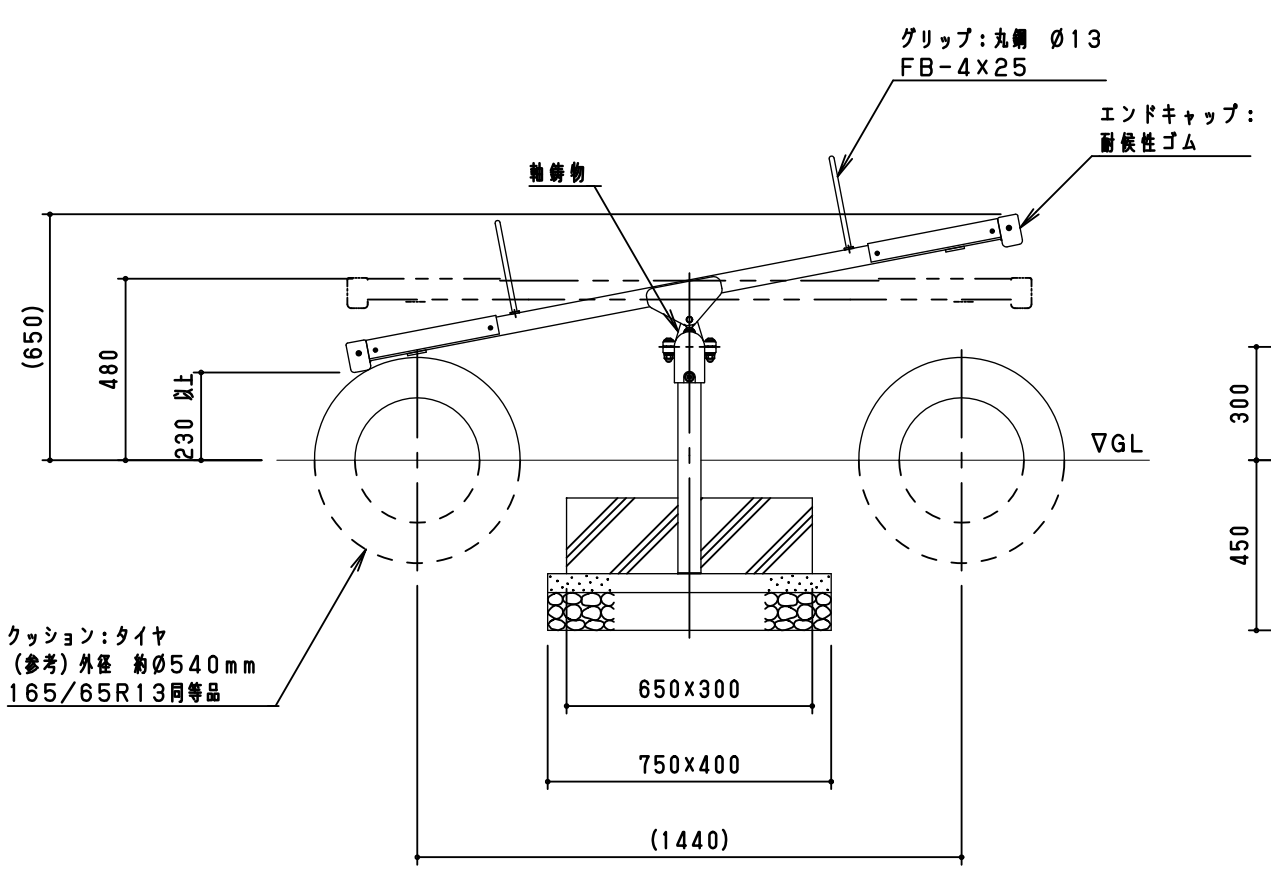
立面図 S = 1 / 20
