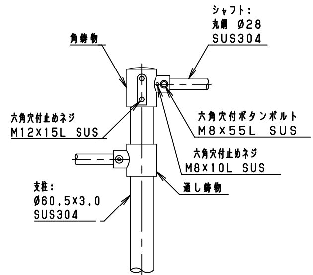
鋳物部／柱脚部詳細図 S = 1 / 10
