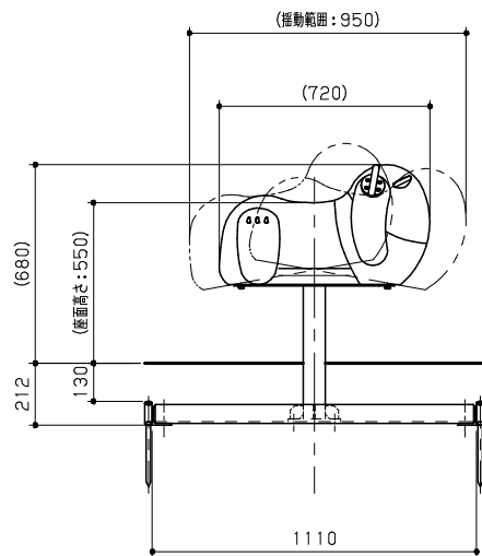
立面図 S = 1 / 20
