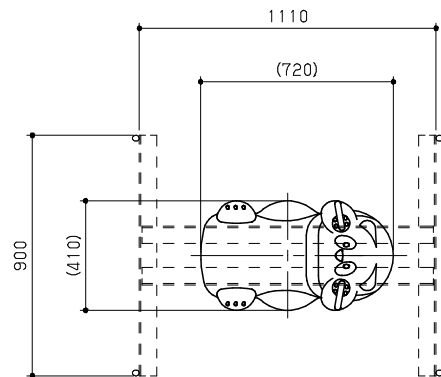
平面図 S = 1 / 20
