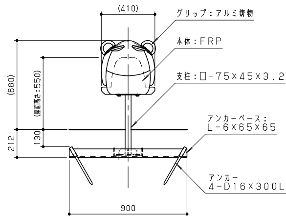
側面図 S = 1 / 20
