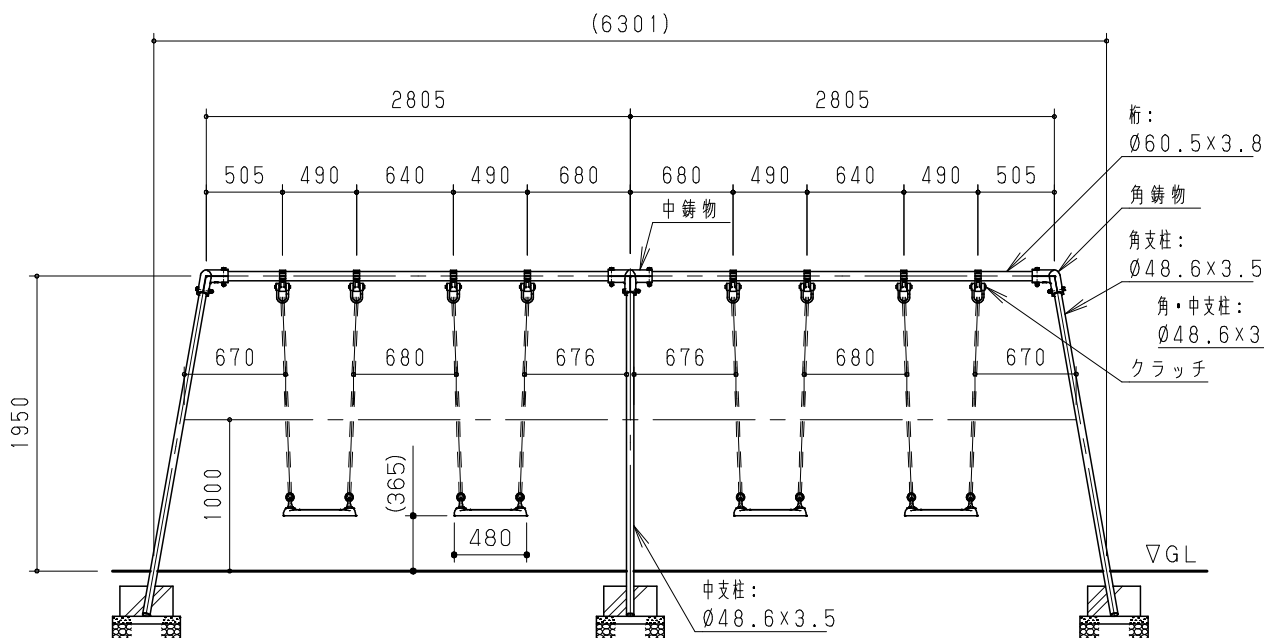
立面図 S = 1 / 50
