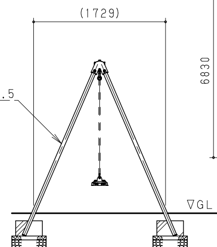
側面図 S = 1 / 50
