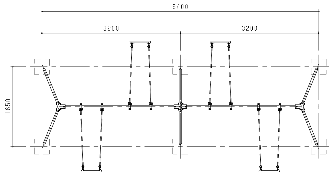
平面図 S = 1 / 50
