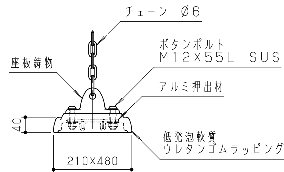
座板詳細図 S = 1 / 10
