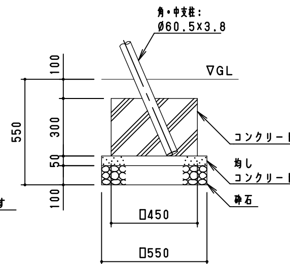
基礎詳細図 S=1/20
