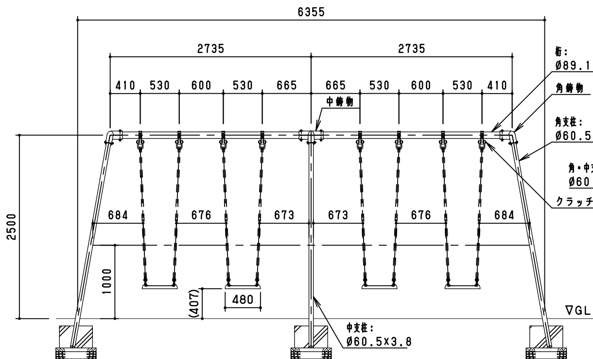
立面図 S=1/50
