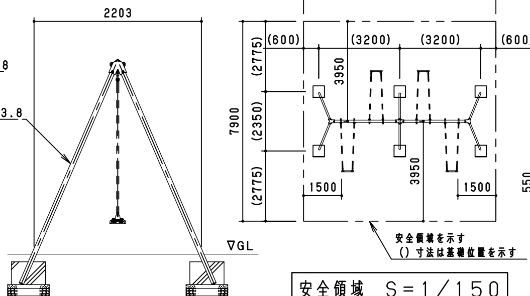
側面図 S=1/50
