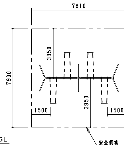
安全領域 S=1/150
