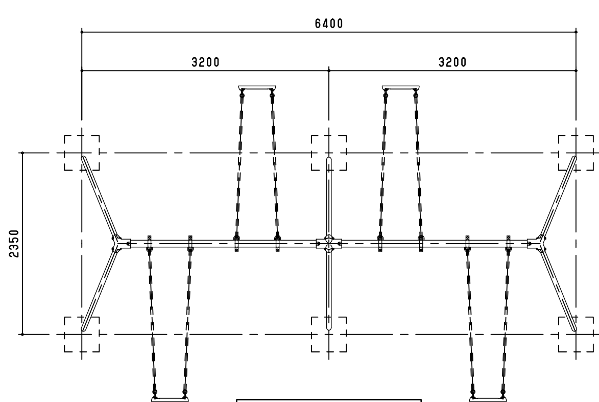
平面図 S=1/50
