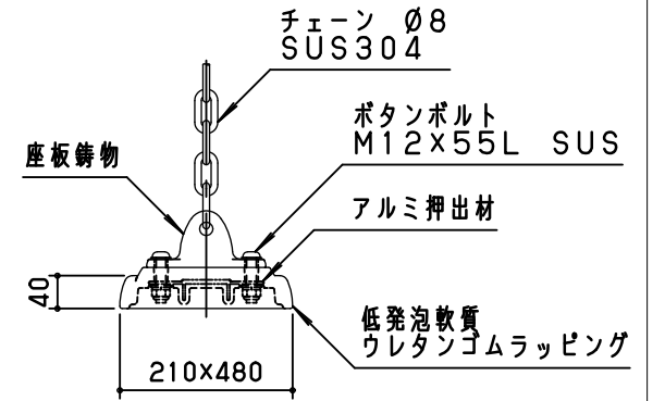
座板詳細図 S=1/10
