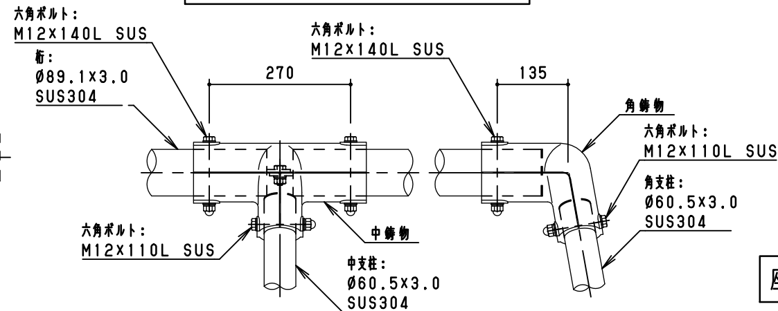
中/角鋳物詳細図 S=1/10
