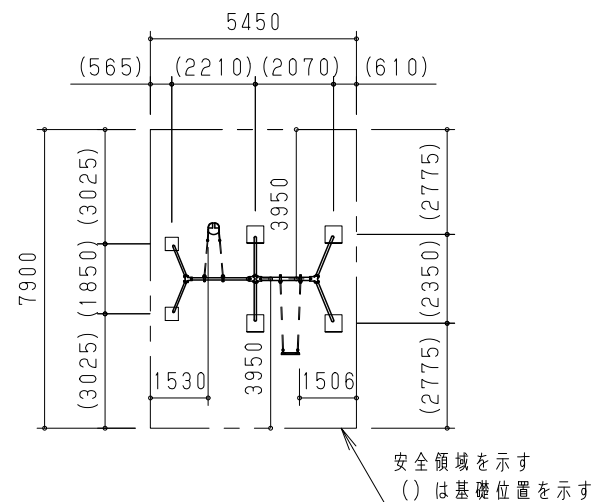
安全領域 S = 1 / 200
