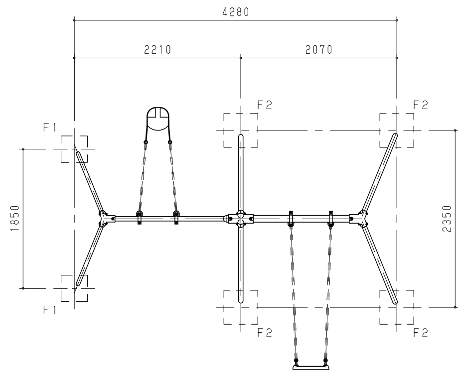
平面図 S = 1 / 50
