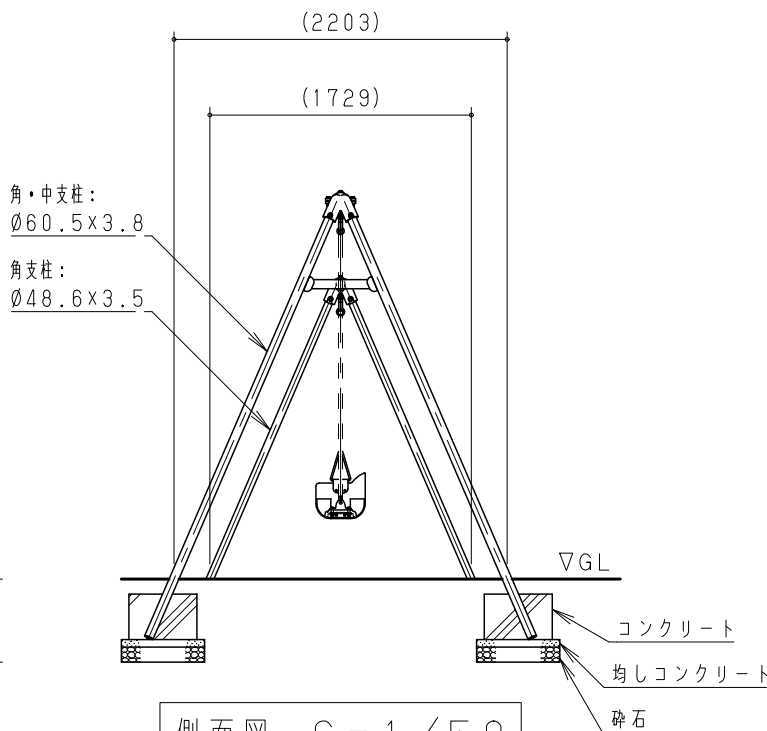
側面図 S = 1 / 50
