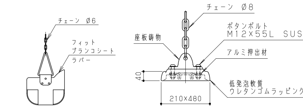
座板1詳細図 S = 1 / 20
