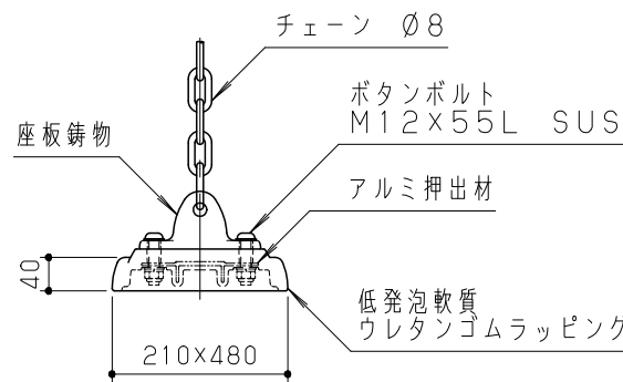
座板2詳細図 S = 1 / 10
