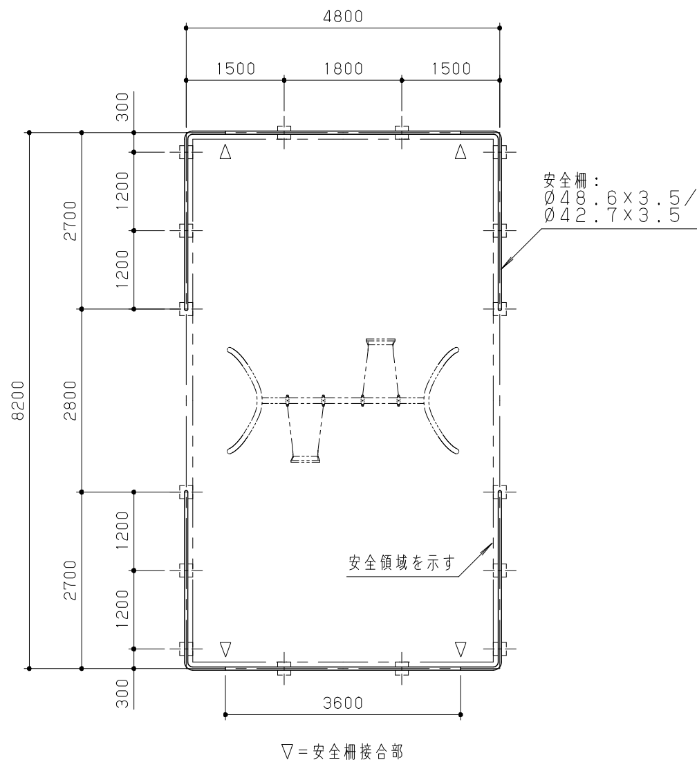
平面図 S = 1 / 80
