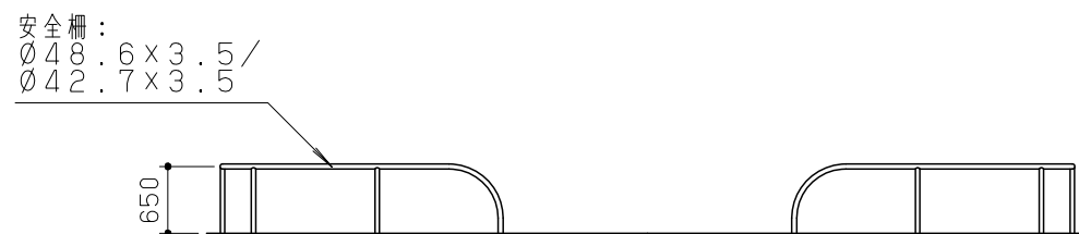
側面図 S = 1 / 80
