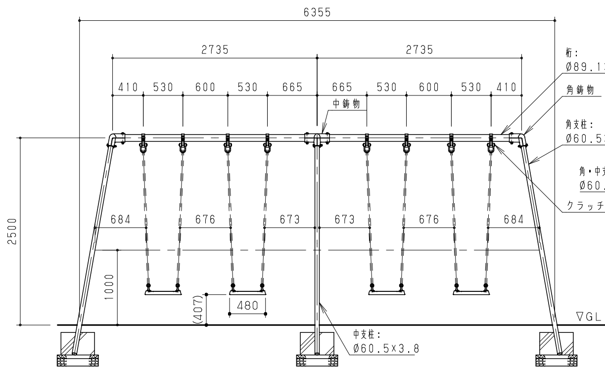
立面図 S = 1 / 50
