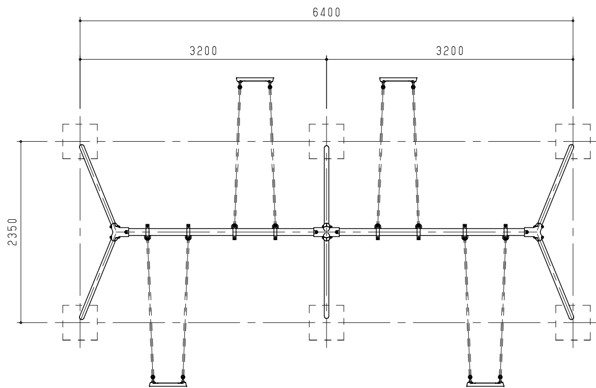
平面図 S = 1 / 50
