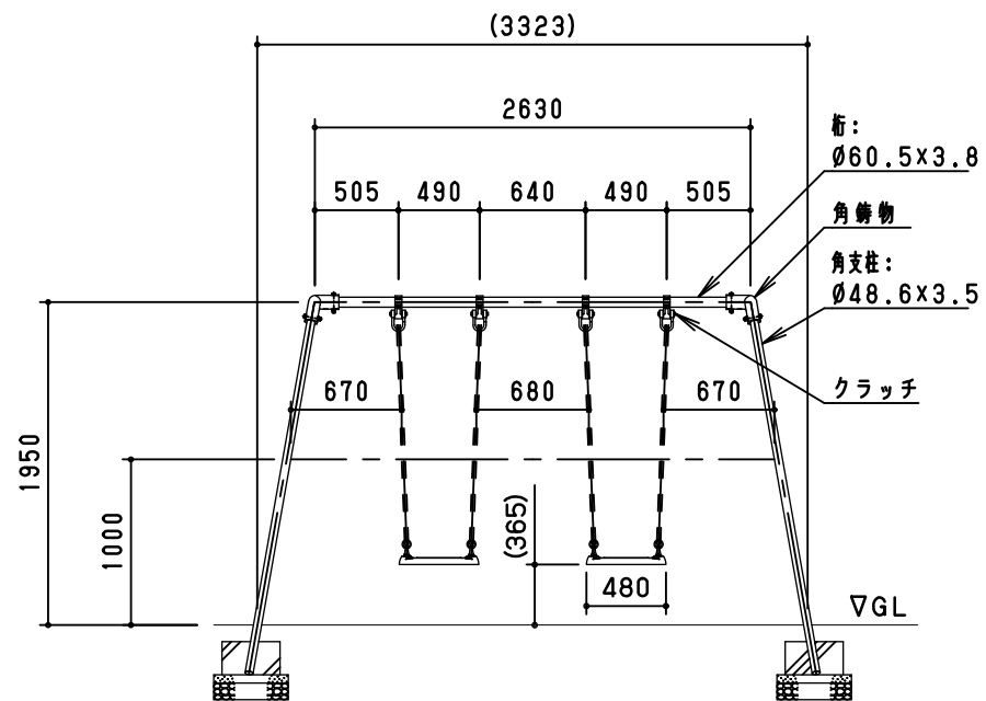
立面図 S=1/50
