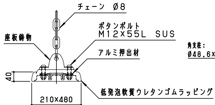
座板詳細図 S=1/10
