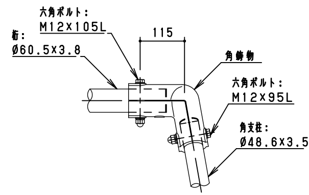
角鋳物詳細図 S=1/10
