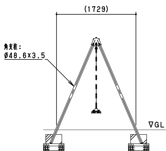
側面図 S=1/50
