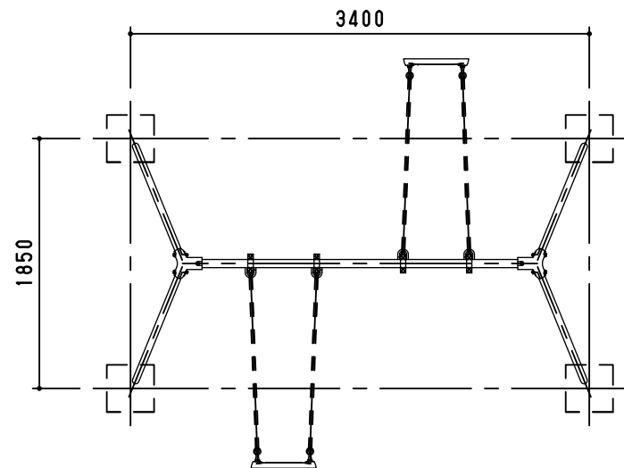
平面図 S=1/50
