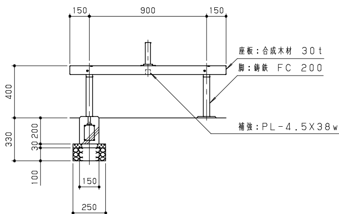
正面図 S=1/20
