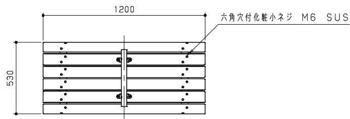
平面図 S=1/20
