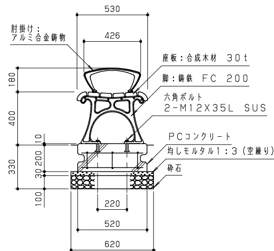
側面図 S=1/20
