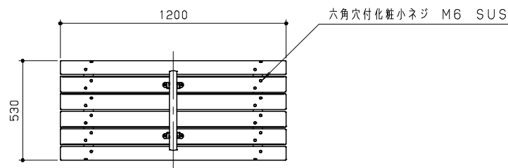
平面図 S=1/20
