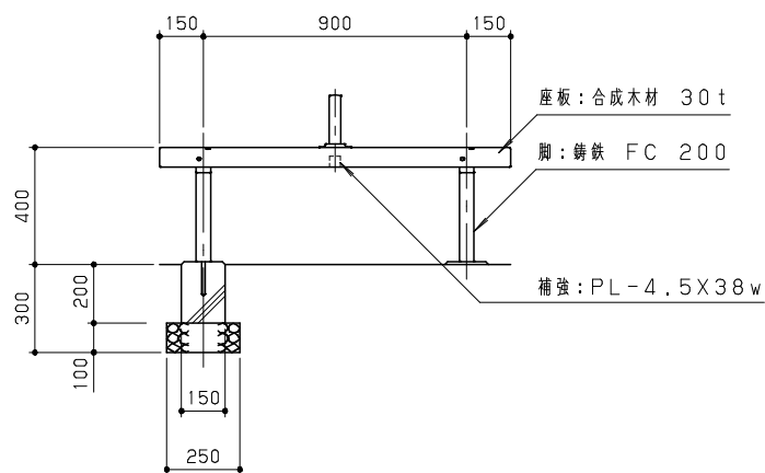
正面図 S=1/20
