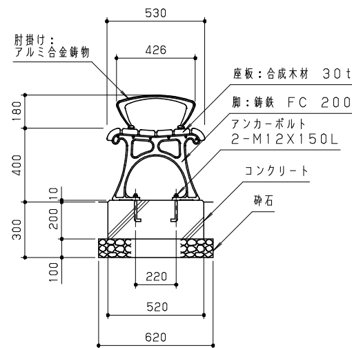
側面図 S=1/20
