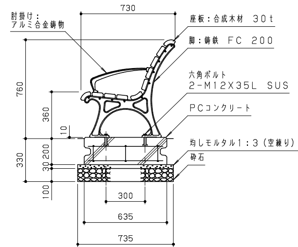
側面図 S = 1 / 20
