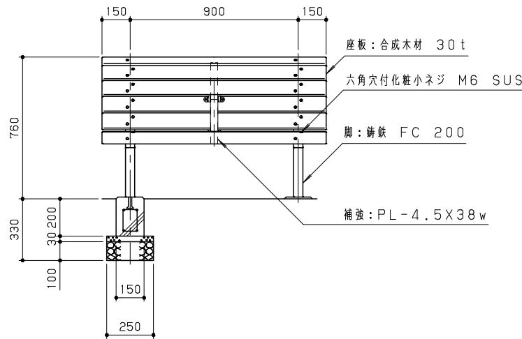
正面図 S = 1 / 20
