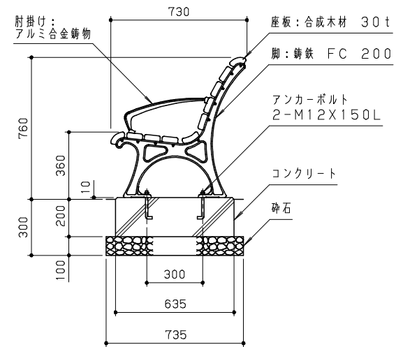
側面図 S = 1 / 20
