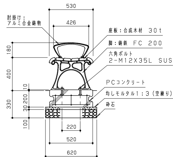
側面図 S=1/20
