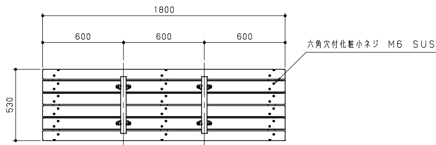
平面図 S=1/20
