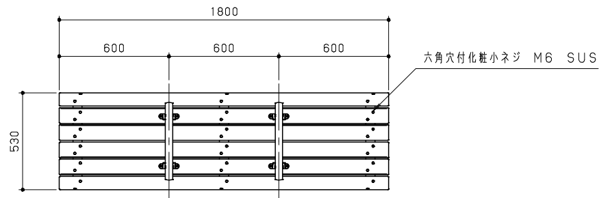
平面図 S=1/20
