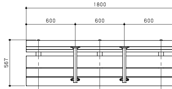
平面図 S = 1 / 20
