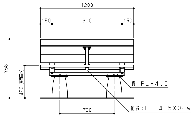
立面図 S = 1 / 20
