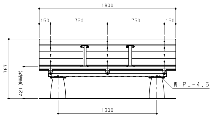
立面図 S = 1 / 20
