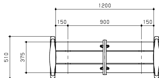
平面図 S = 1 / 20
