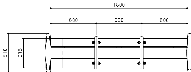
平面図 S=1/20
