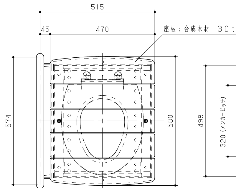
平面図 S=1/10
