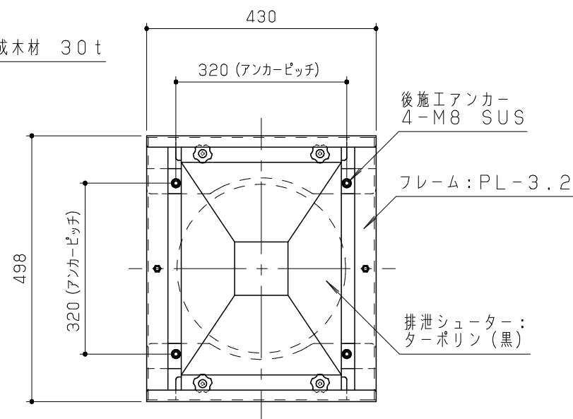
平面図 S=1/10
