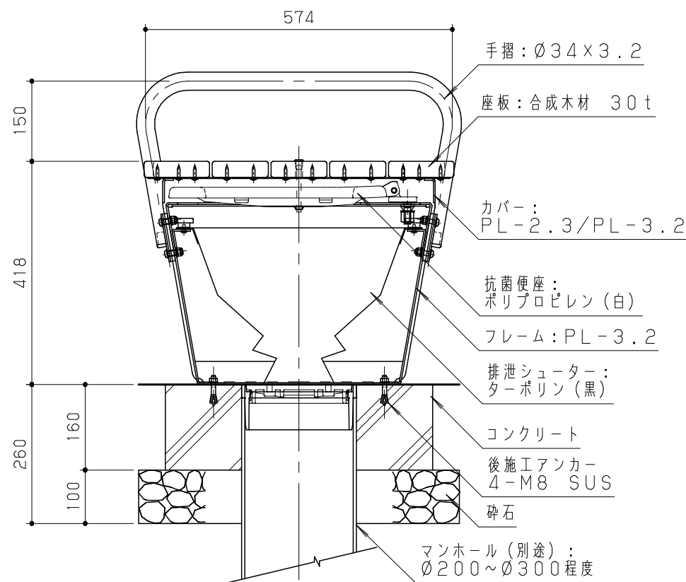
側断面図 S=1/10
