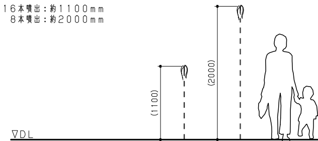
噴水姿図 (概略) S = 1 / 40
