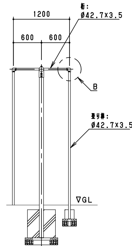
側面図 S=1/50
