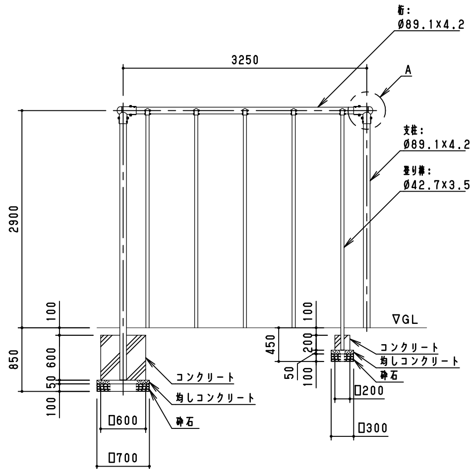
平面図 S=1/50
