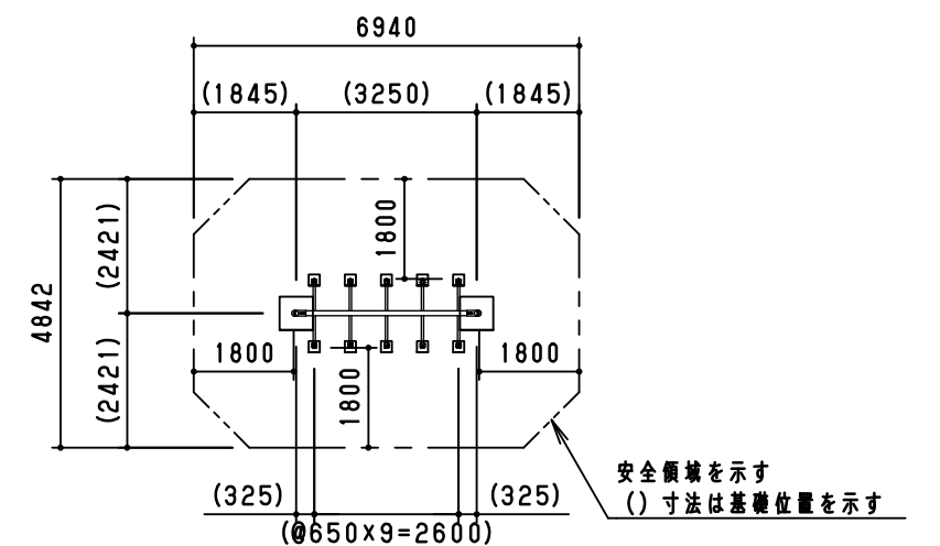
安全領域 S=1/150
