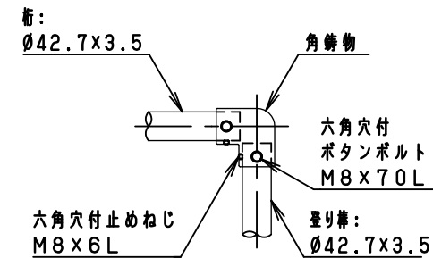
B詳細図 S=1/10
