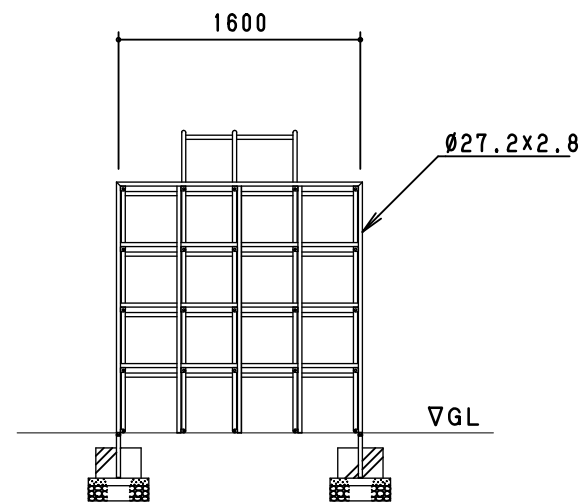
側面図 S = 1 / 50
