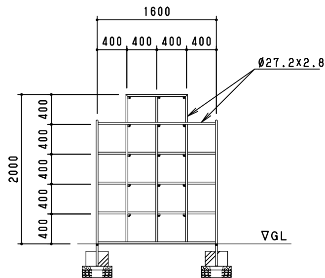
立面図 S = 1 / 50
