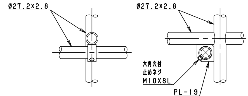
止めネジジョイント部
