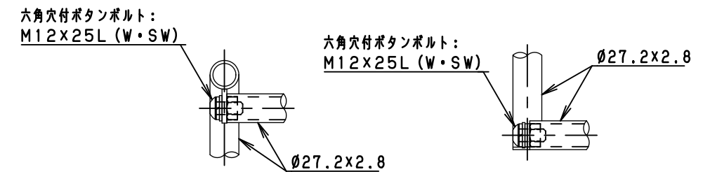
パネル接続部
