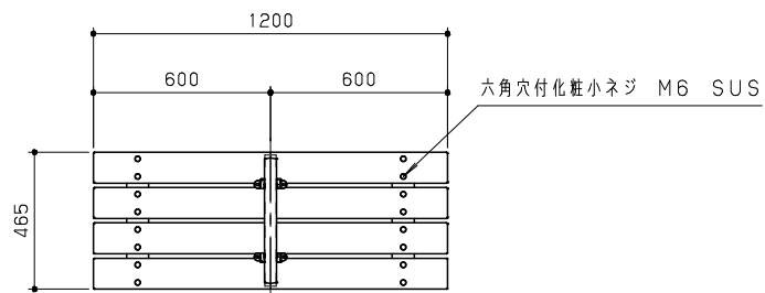
平面図 S = 1 / 20
