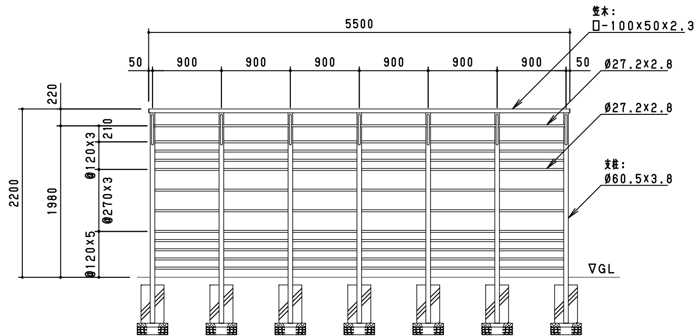
正面図 S=1/50
