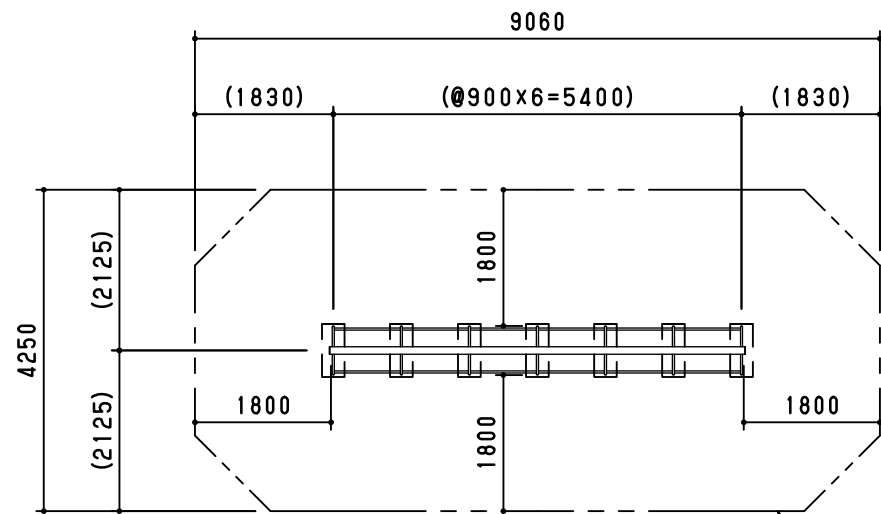
安全領域 S=1/100
