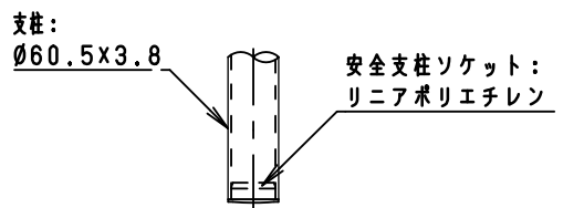
柱脚部詳細図 S=1/10
