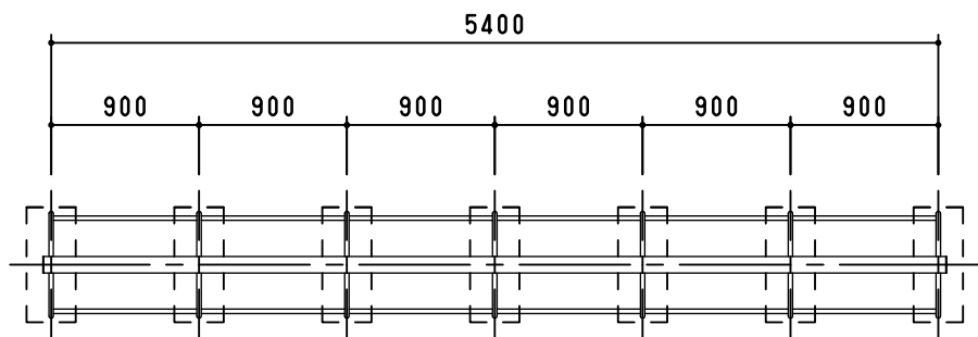
平面図 S=1/50
