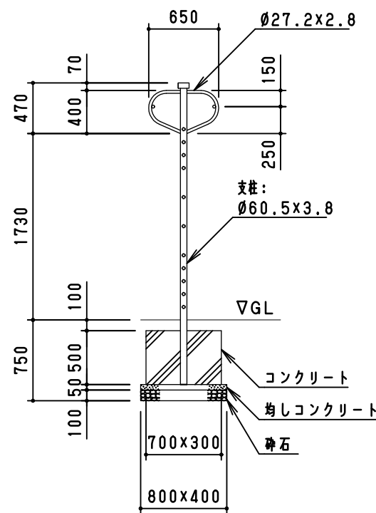
側面図 S=1/50
