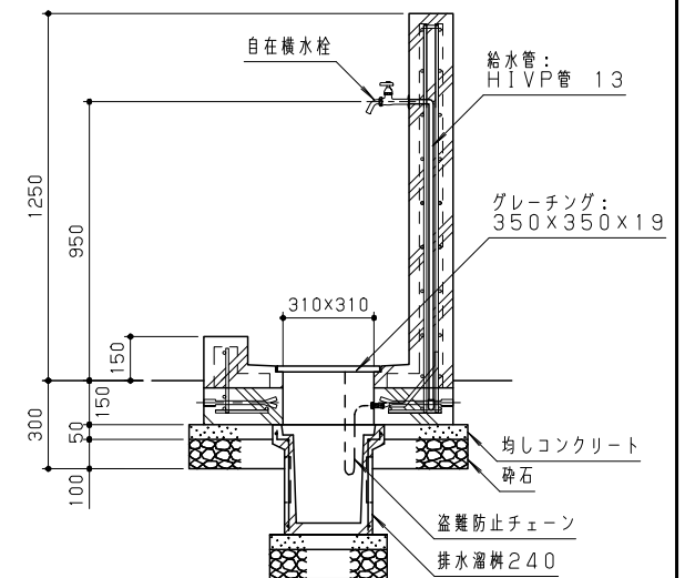
断面図 S=1/20
