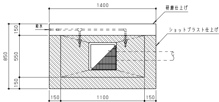
平面図 S=1/20
