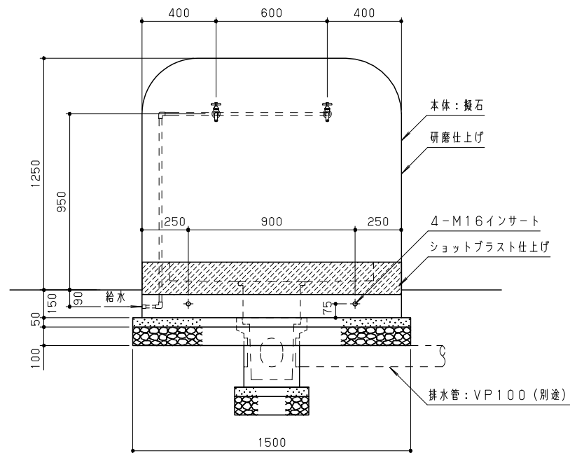
立面図 S=1/20
