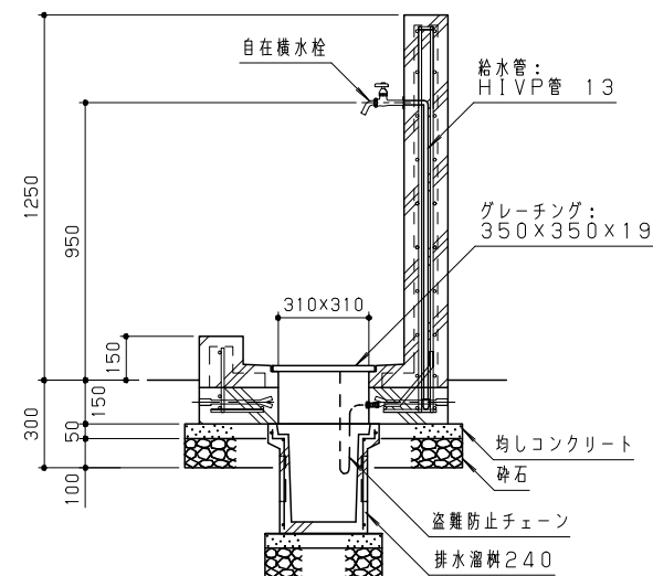
断面図 S = 1 / 20
