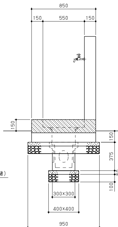
側面図 S = 1 / 20
