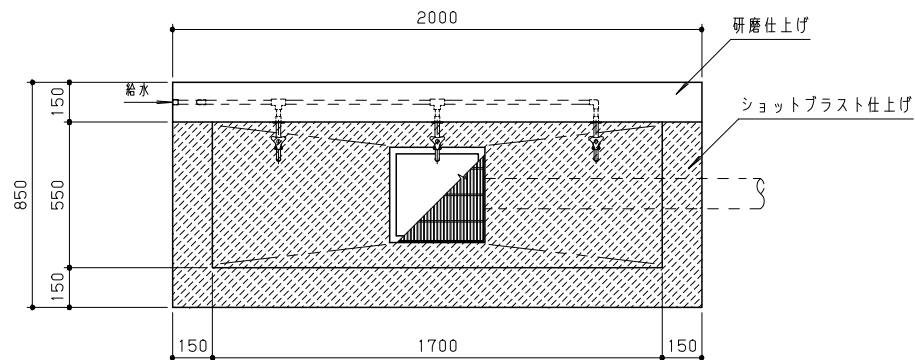
平面図 S = 1 / 20
