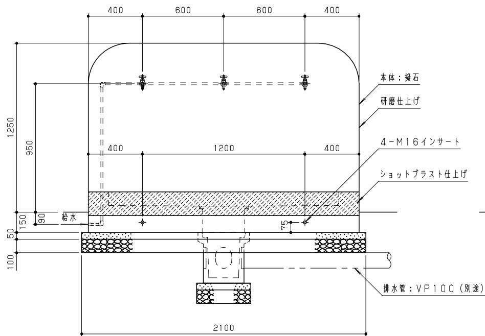
立面図 S = 1 / 20
