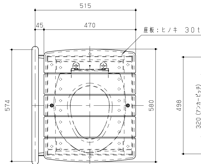
平面図 S = 1 / 10
