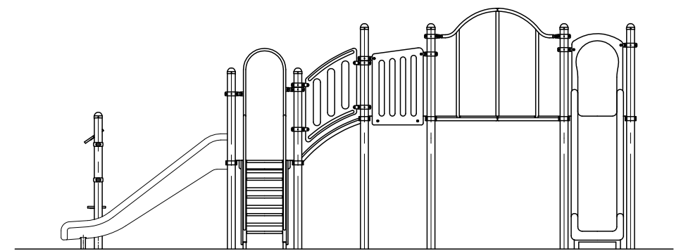
B 視 立 面 図 S = 1 / 6 0
